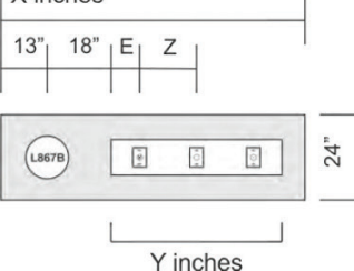
3 Module
